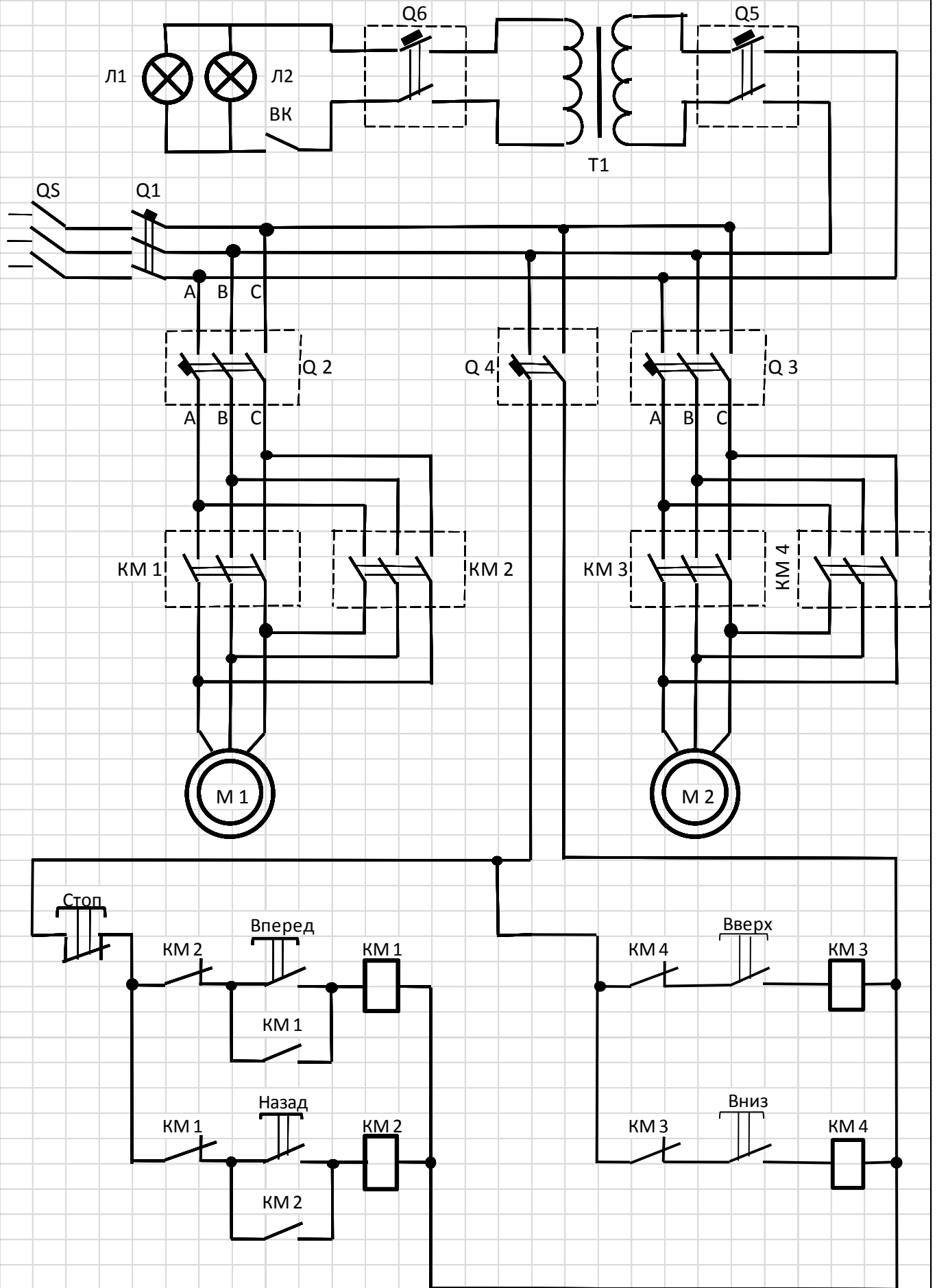
Схема электрическая принципиальная Станка БУ - 20 - 2 АМ Рис. 12
