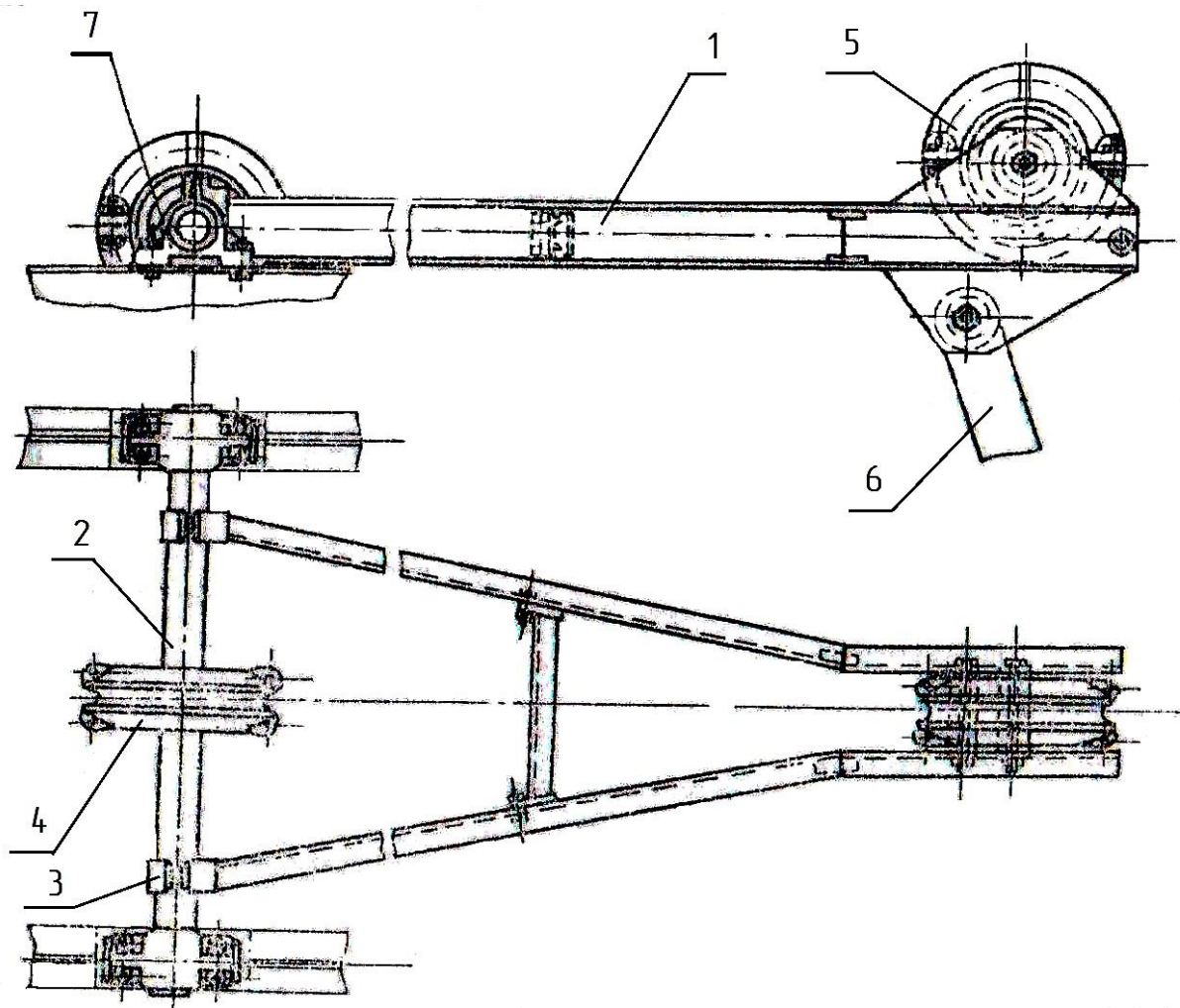
Рис. 3 Ударная балка
