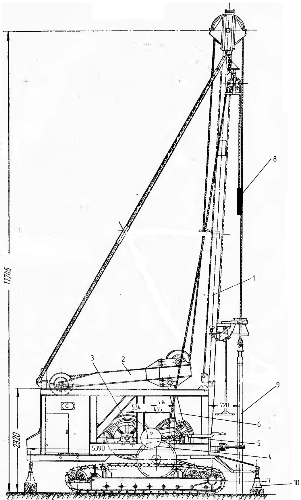
Буровой станок БУ-20-2 АМ
