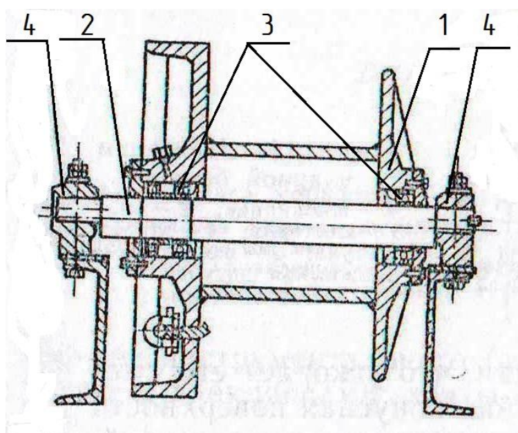
Рис 5. Лебедка подъема желонки
