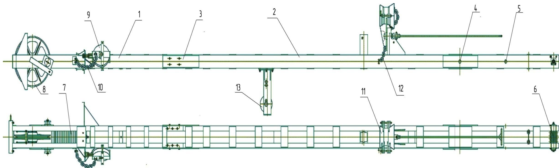
Рис 2. Стрела
