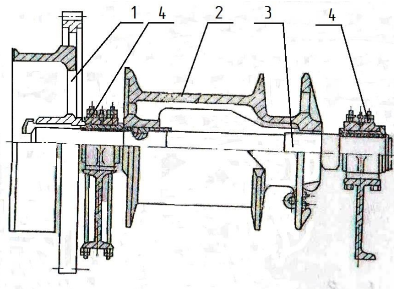
Рис 4. Инструментальная лебедка
