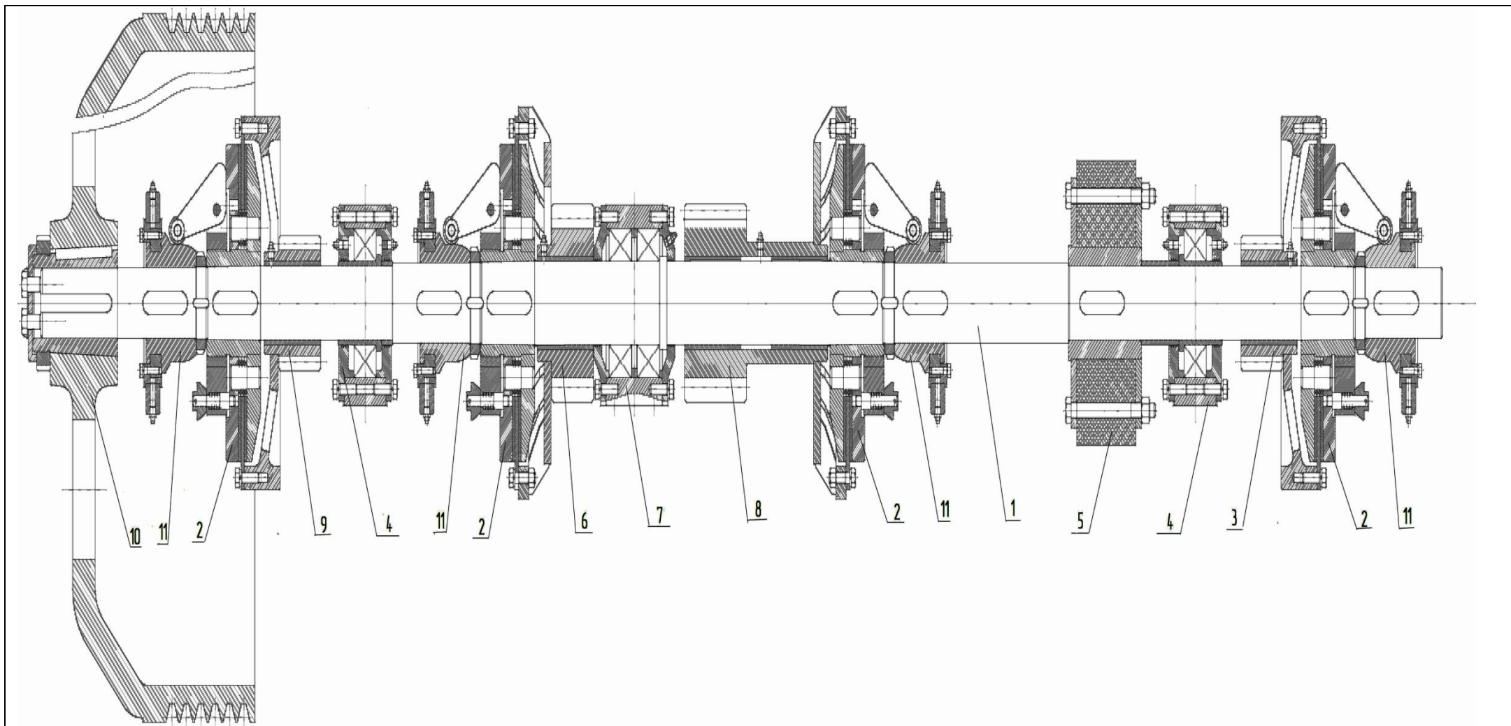
Рис 8. Вал главный
