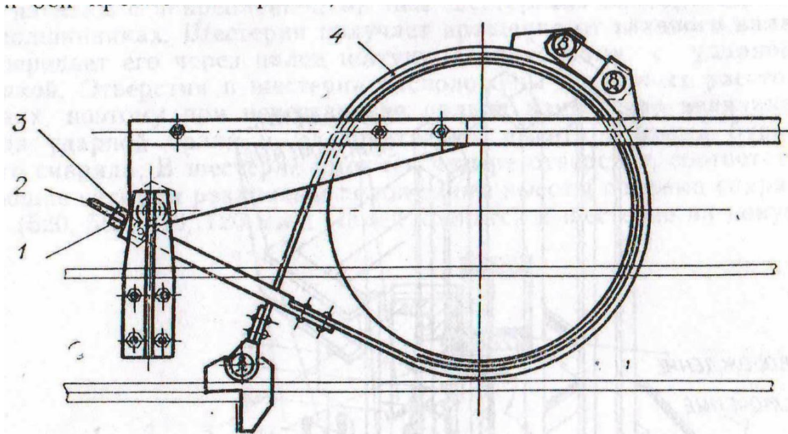
Рис. 10. Регулировка тормоза инструментального барабана.
