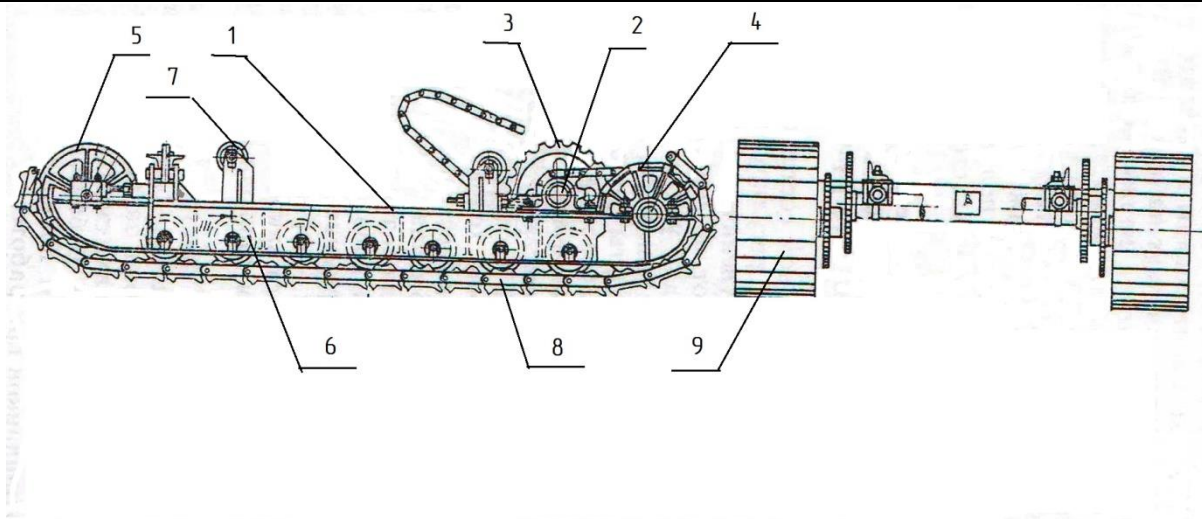
Рис. 7 Ход гусеничный
